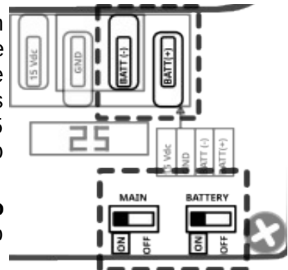
Ilustración 7: Conectores de batería y Switches de corte de alimentación
