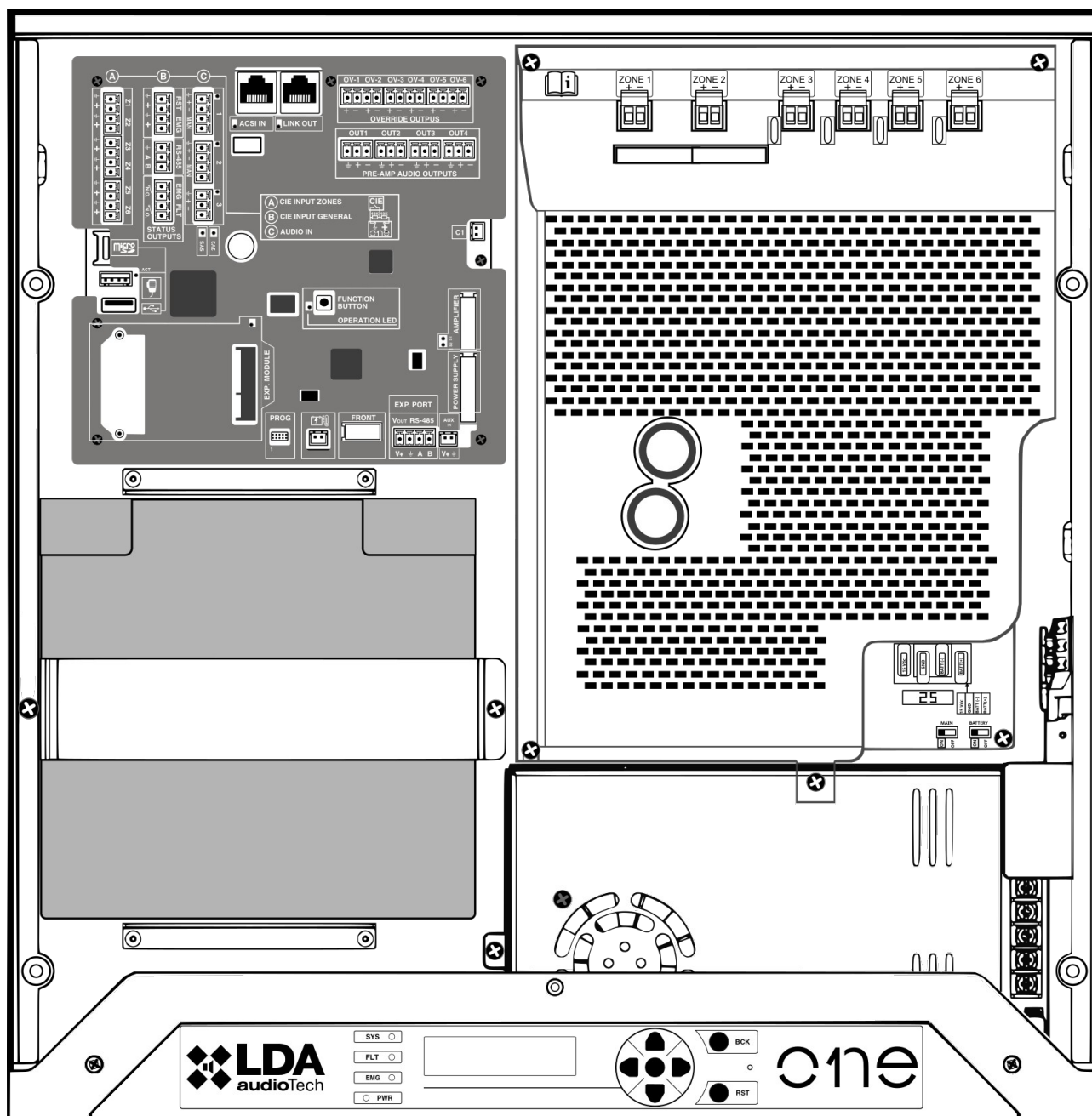
Ilustración 2: Vista interior
