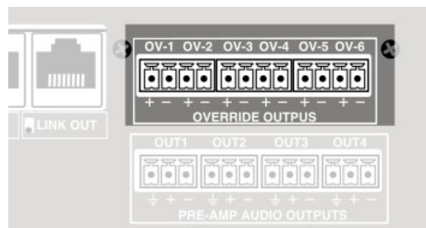
Ilustración 18: Salida Anulación Atenuadores
