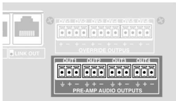
Ilustración 17: Salidas preamplificadas
