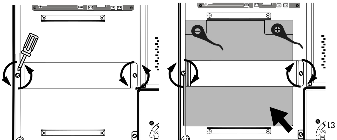
Ilustración 8: Instalación de la batería
