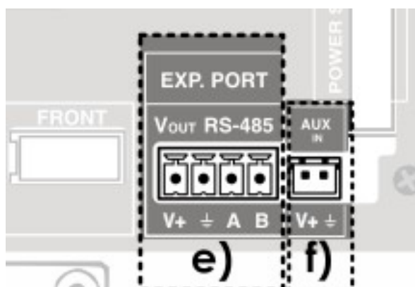
Ilustración 20: Otras conexiones internas
