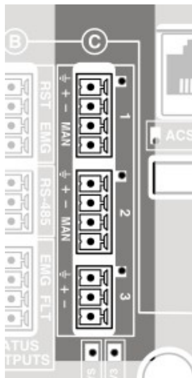
Ilustración 12: Entradas Fuente de Audio
