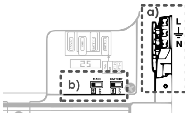
Ilustración 6: a) Conexiones de Alimentación
