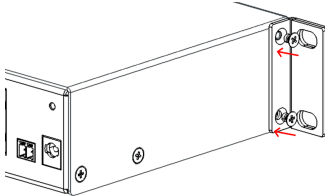
Ilustración 16: Montaje escuadra de fijación corta
