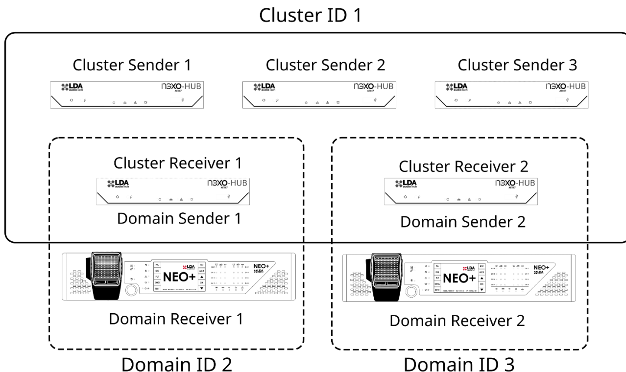
Ilustración 24: Sistema ACSiNet
