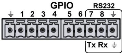
Ilustración 5: Puertos de integración
