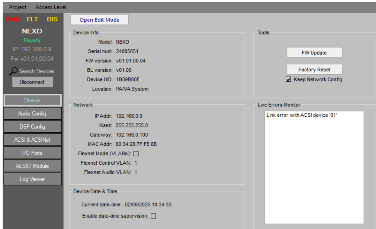
Ilustración 29: Interfaz NEXO Config Tool
