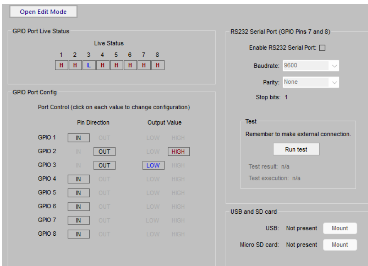
Ilustración 51: I/O Ports
