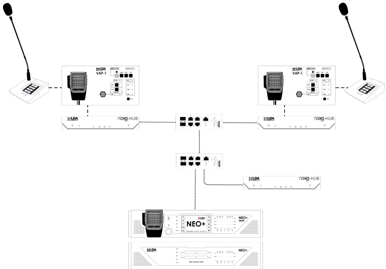
Ilustración 26: Cluster ACSI Net
