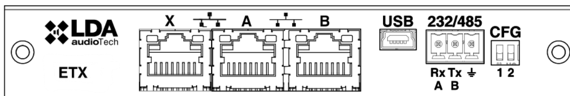
Ilustración 1: Bahía ETX de conexión a sistema
