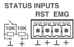
Ilustración 10: Entrada activación de emergencia general
