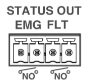
Ilustración 11: Salidas estado sistema
