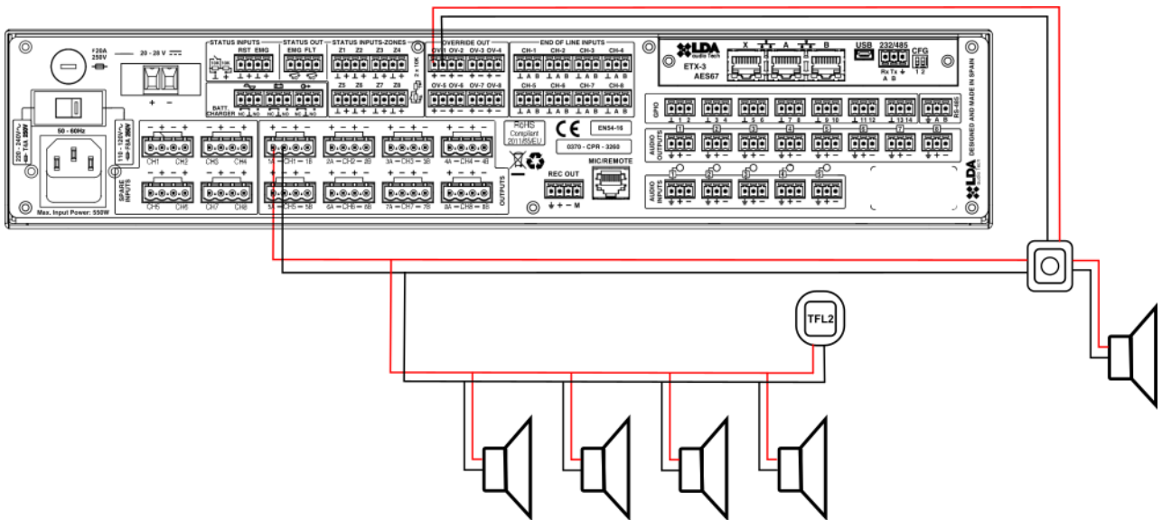
Ilustración 39: Conexión controlador de volumen
