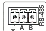
Ilustración 31: Bus serie ECI
