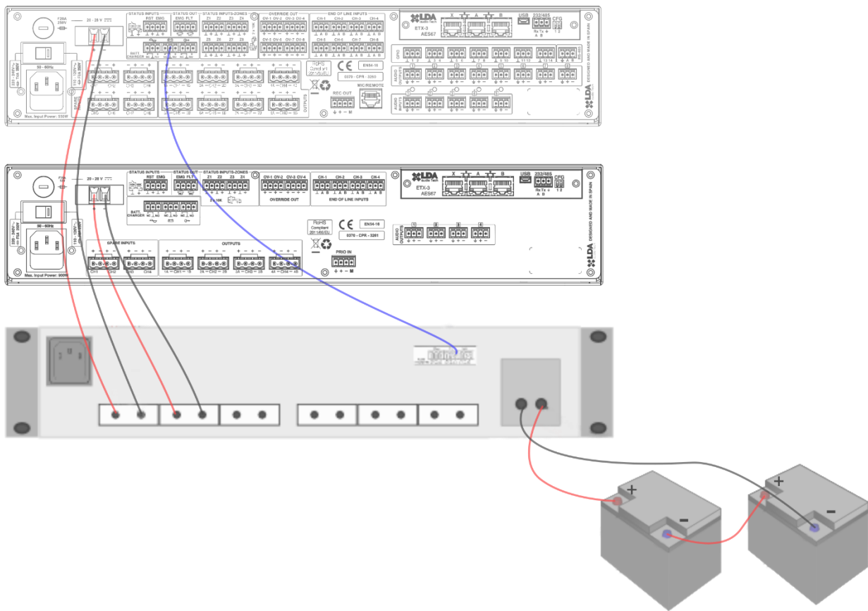
Ilustración 32: Esquema alimentación emergencia
