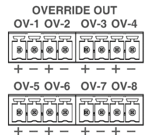
Ilustración 13: Salida anulación atenuadores
