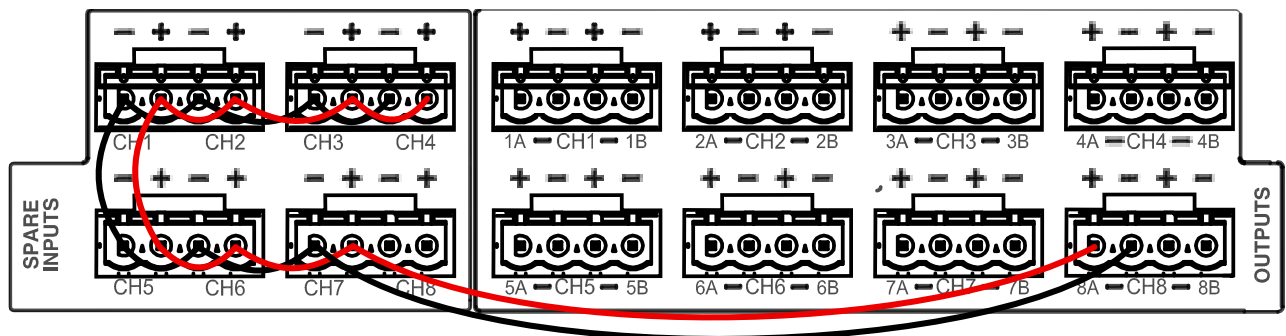
Ilustración 40: Conexión amplificador de reserva
