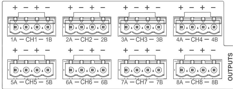
Ilustración 23: Salidas líneas de altavoces
