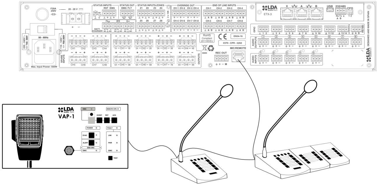
Ilustración 33: Conexión micrófonos y dispositivos ACSI
