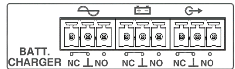
Ilustración 7: Entradas monitor alimentación emergencia
