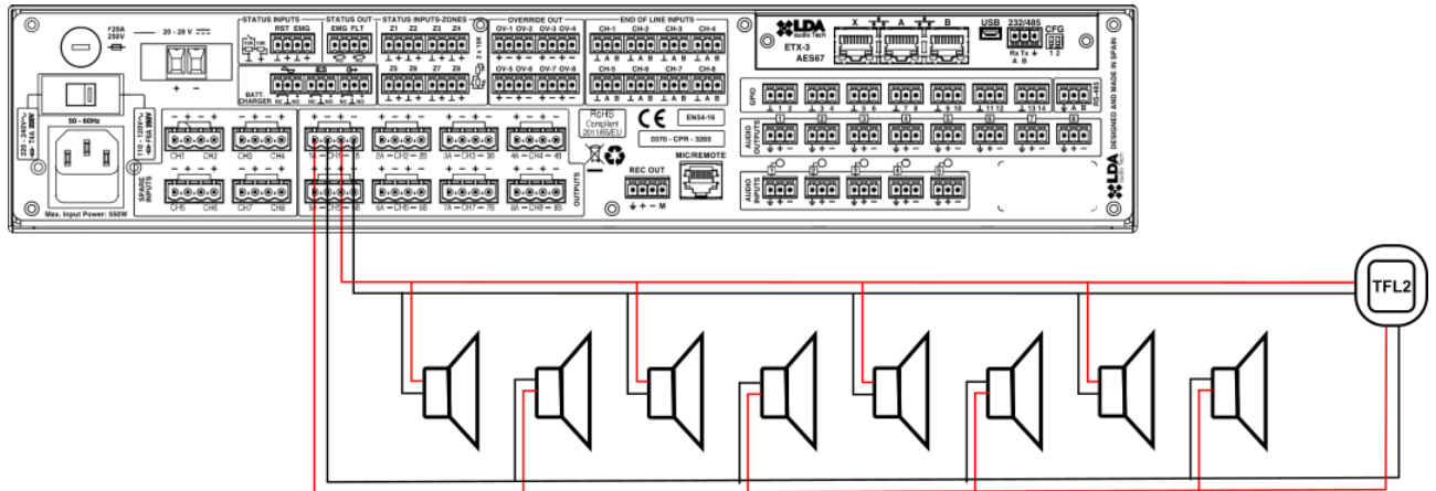
Ilustración 37: Línea de altavoces. Modo Clase-A
