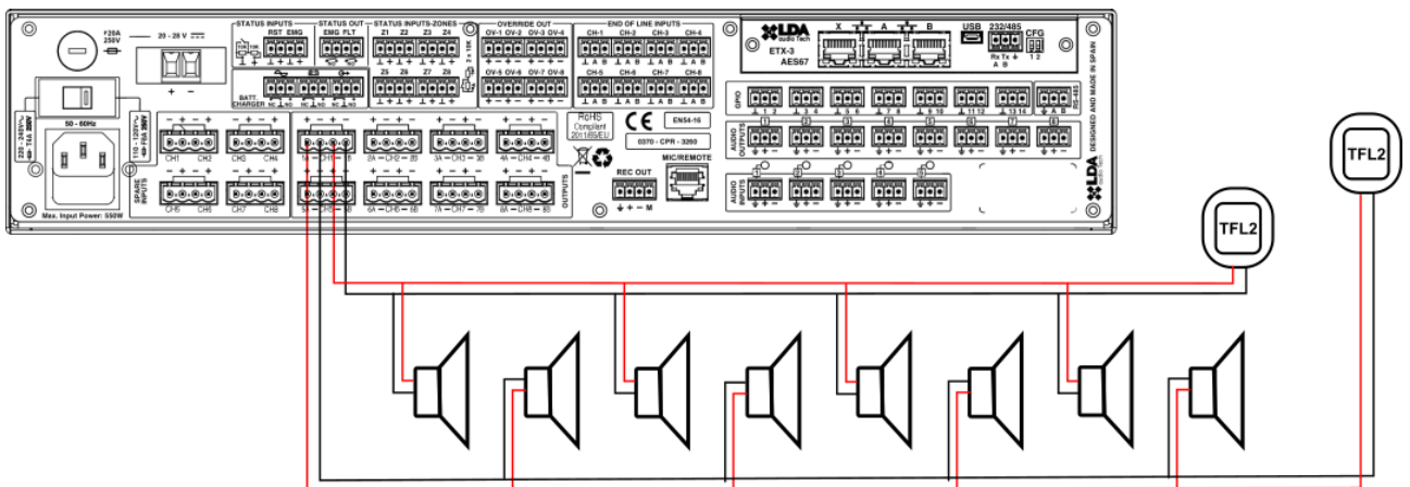
Ilustración 36: Líneas de altavoces. Modo AB
