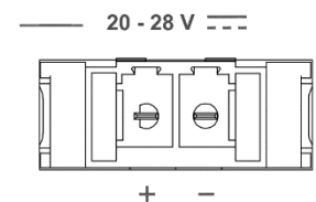
Ilustración 21: Entrada alimentación emergencia
