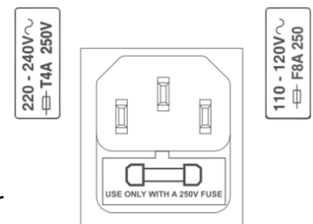
Ilustración 20: Fusible alimentación principal
