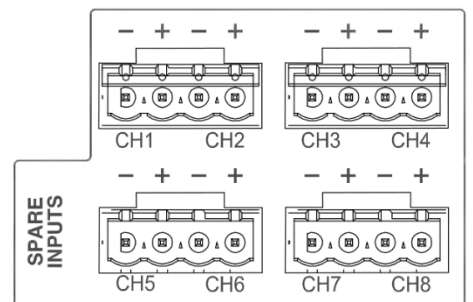
Ilustración 24: Entradas amplificadores de reserva
