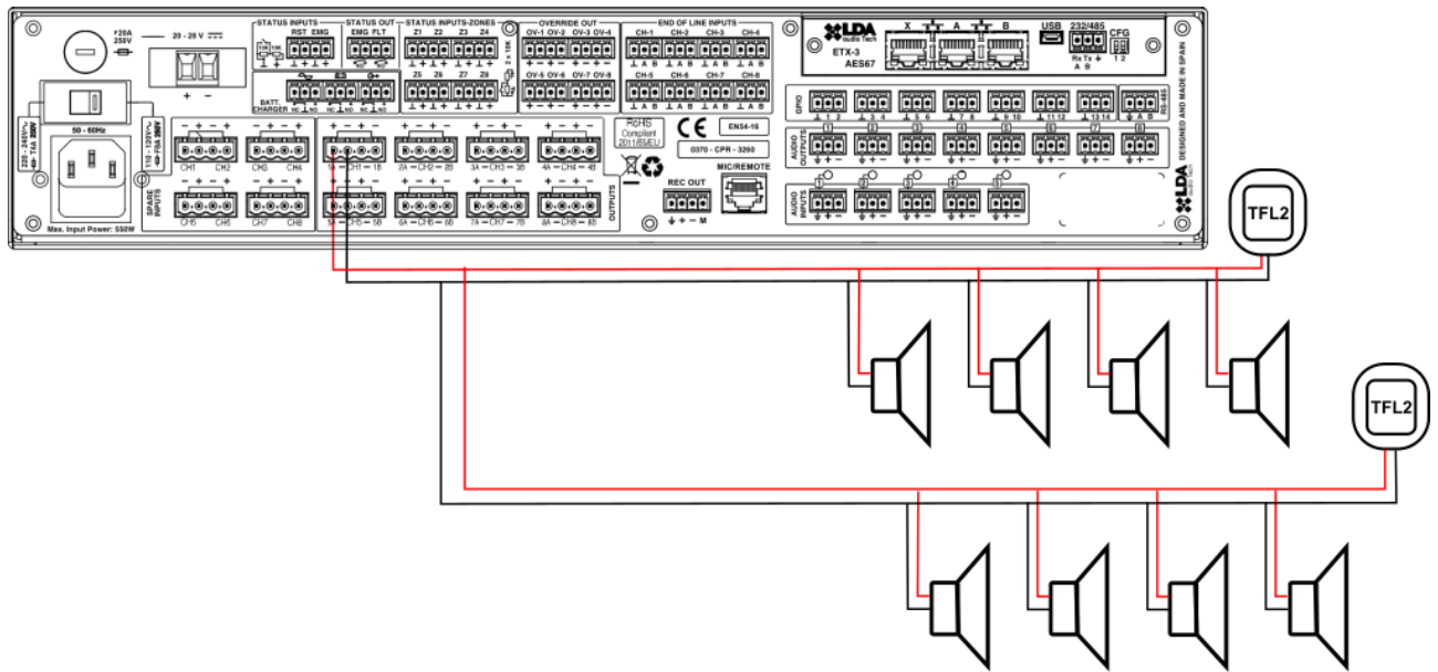
Ilustración 38: Conexión de Terminadores de línea de altavoces
