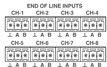
Ilustración 14: Entradas terminadores de línea de altavoces
