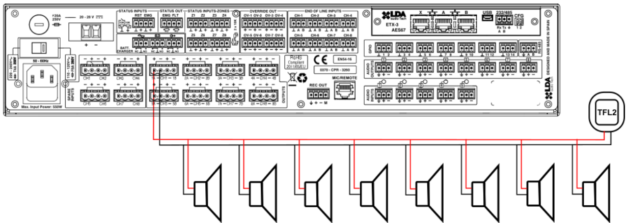
Ilustración 35: Líneas de altavoces. Modo estándar
