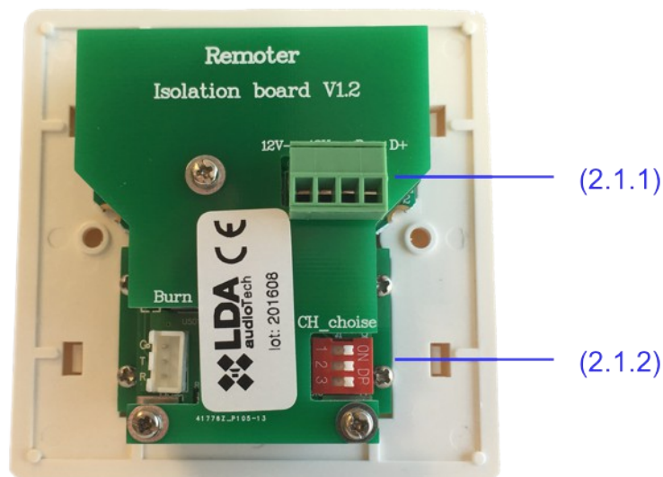
Ilustración 1: Trasera VCC-64
