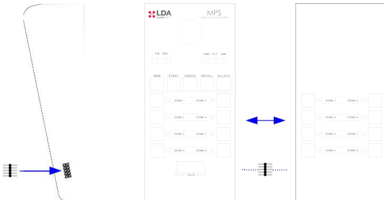
Ilustración 7: Instalación Extensiones Teclado MPS-8K
