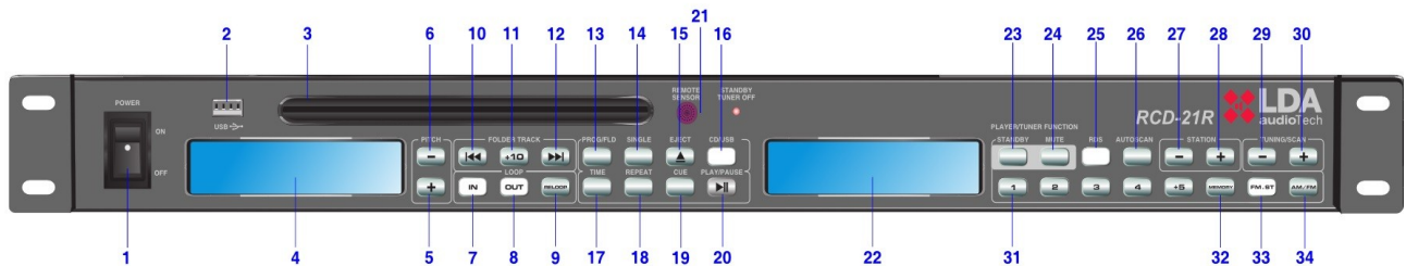
Ilustración 1: Panel Frontal
