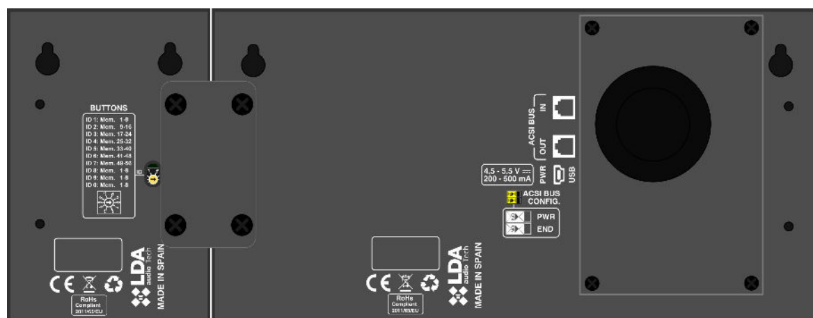
Ilustración 14: Conexión Teclado Expansión. Paso 4 Bloqueo
