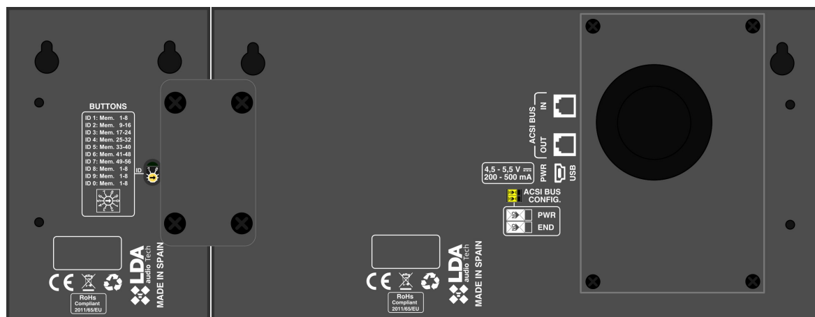
Ilustración 14: Conexión Teclado Expansión. Paso 4 Bloqueo
