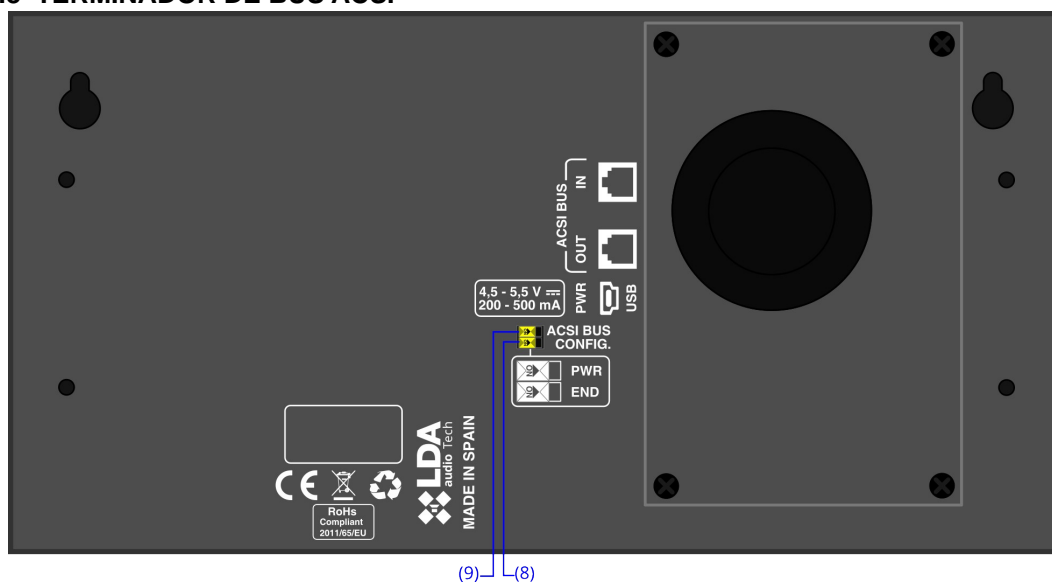
Ilustración 3: Selectores BUS ACSI
